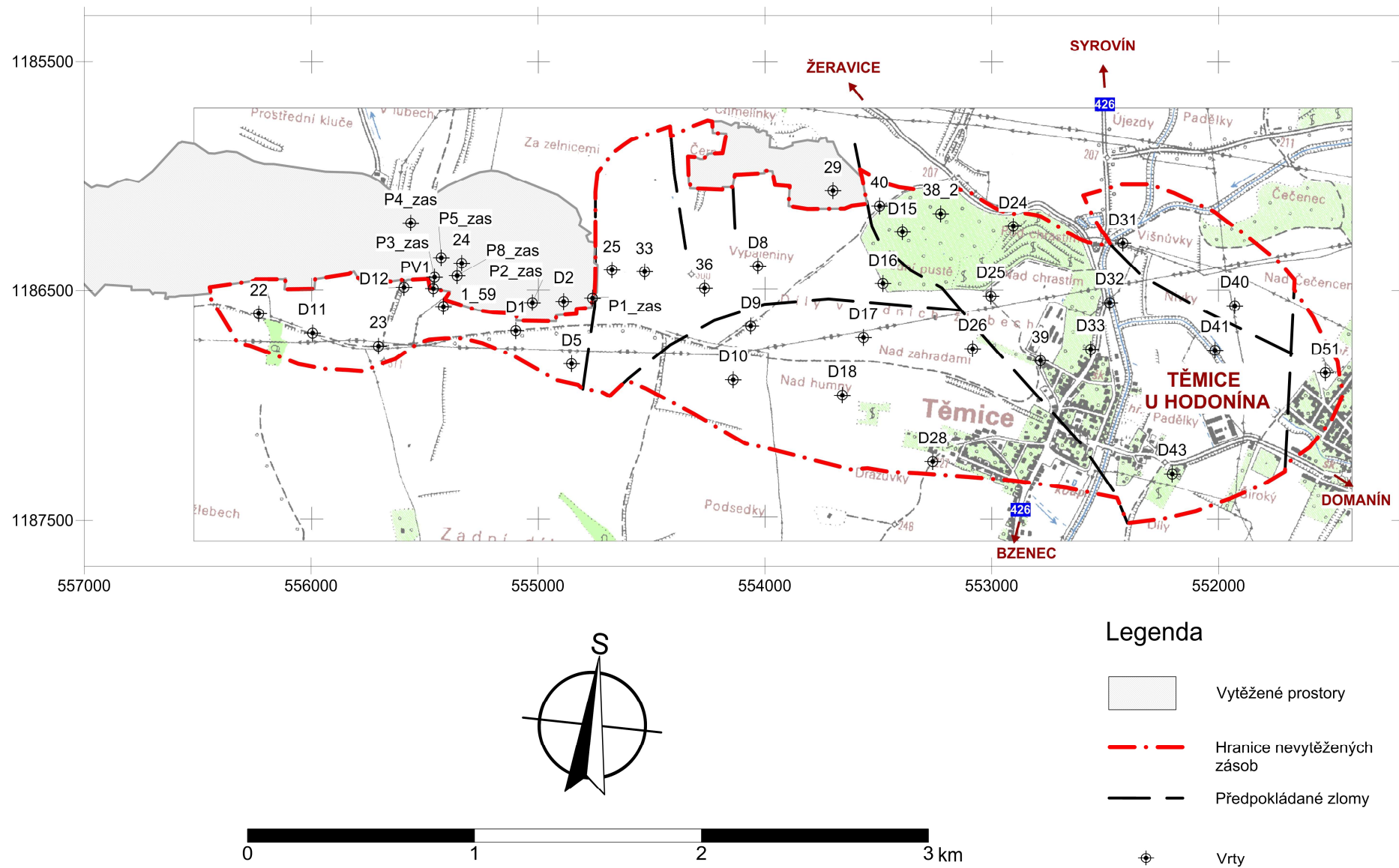
Obr. 2: Pozice vrtů, vytěžených prostor a oblastí nevytěžených zásob zpracovávané oblasti nad topografickou mapou.
